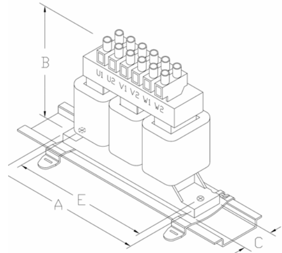
Figure 2 35mm DIN Mount option
